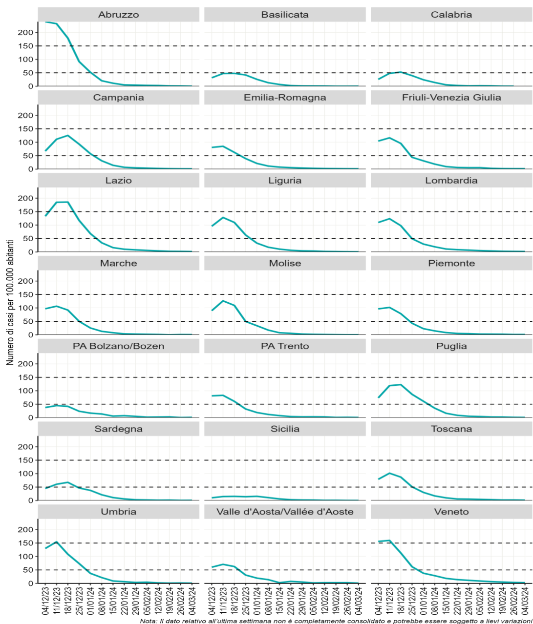
Figura 18 - Incidenza settimanale di diagnosi di infezioni per SARS-CoV-2 (per 100.000 ab.) per Regione/PPAA dal 4 dicembre 2023
