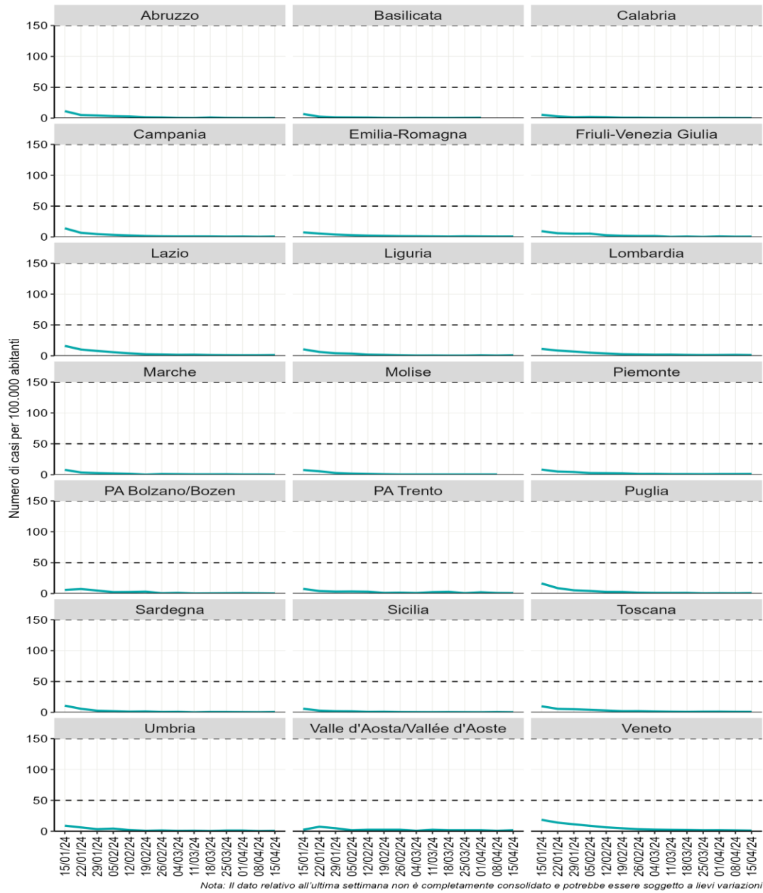
Figura 18 - Incidenza settimanale di diagnosi di infezioni per SARS-CoV-2 (per 100.000 ab.) per Regione/PPAA dal 15 gennaio 2024
