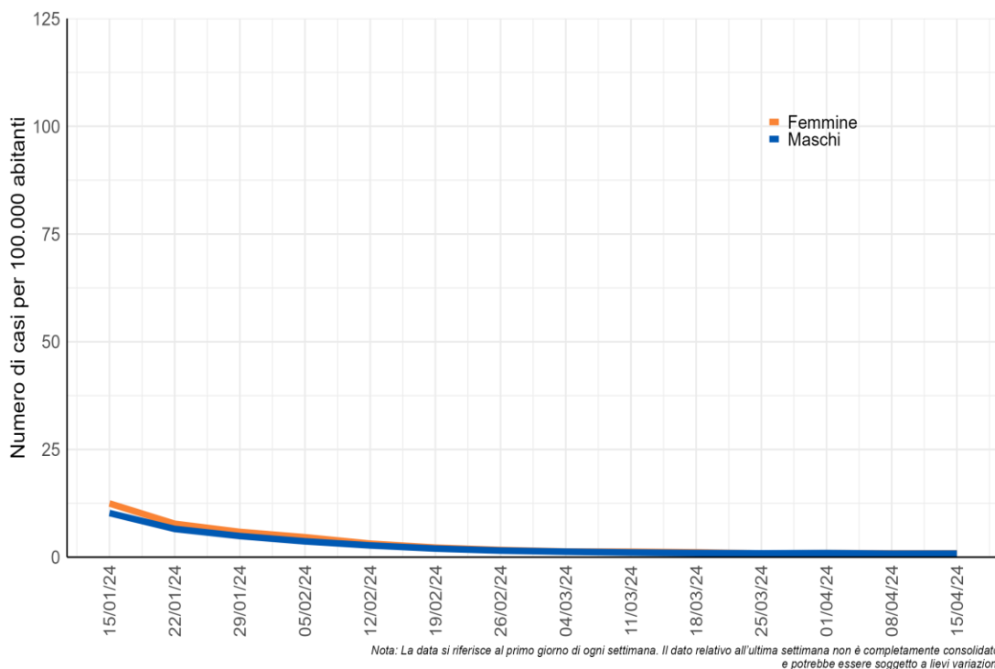
Figura 3 - Incidenza settimanale di diagnosi di infezione da SARS-CoV-2 per 100.000 abitanti per sesso a partire dal 15 gennaio 2024
