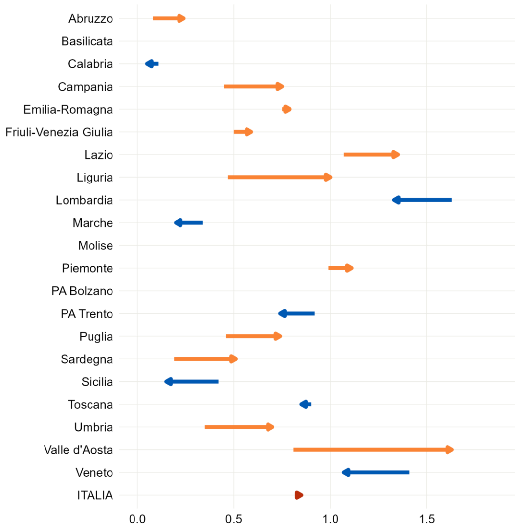
Figura 7 - Andamento dell'incidenza (per 100.000 ab.) per Regione/PA di infezioni da SARS-CoV-2 segnalate nel periodo 15 - 21/04/2024 rispetto a quella nel periodo 08 - 14/04/2024
