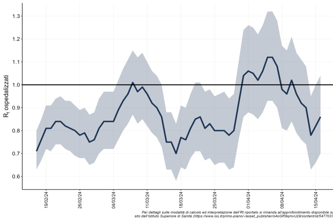
Figura 8 - Andamento giornaliero di Rt ospedalizzazioni nazionale, calcolato con dati estratti il 24 aprile 2024
