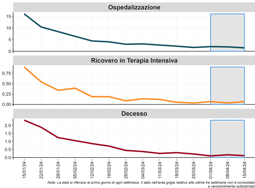
Figura 12 - Tasso settimanale di ospedalizzazione, ricovero in terapia intensiva e decesso in pazienti con diagnosi di infezione da SARS-CoV-2 (per 1.000.000 ab.), a partire dal 15 gennaio 2024
