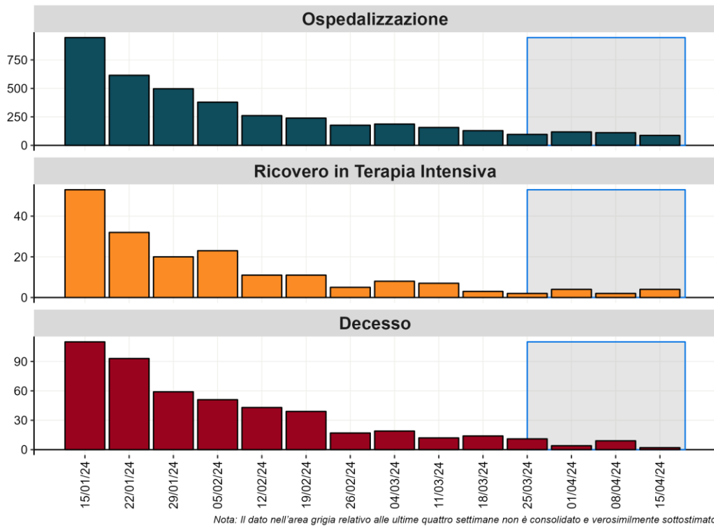
Figura 11 - Numero settimanale di ospedalizzazioni, ricoveri in terapia e decessi per settimana dell'evento a partire dal 15 gennaio 2024
