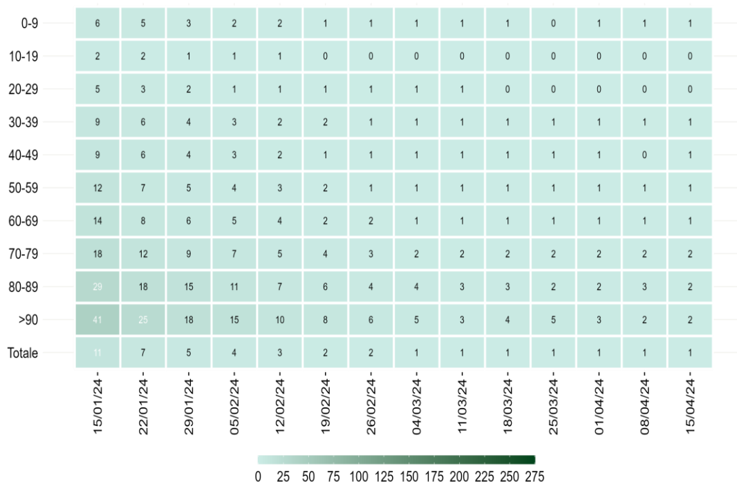
Figura 4 - Incidenza settimanale di infezioni da SARS-CoV-2 per 100.000 abitanti per fascia d'età, a partire dal 15 gennaio 2024
