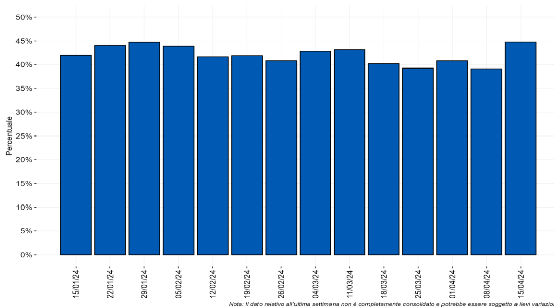
Figura 9 - Distribuzione percentuale settimanale delle diagnosi di reinfezione da SARS-CoV-2 sul totale delle diagnosi segnalate per data di prelievo/diagnosi a partire dal 15 gennaio 2024
