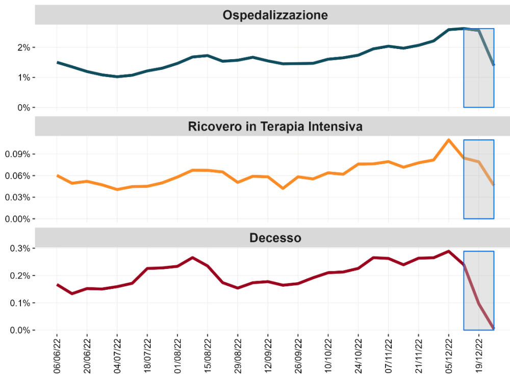
FIGURA 3 - PERCENTUALE SETTIMANALE DI INFEZIONI DA SARS-CoV-2 CON ESITO GRAVE (OSPEDALIZZAZIONE, RICOVERO IN TI E DECESSO), PER SETTIMANA PRELIEVO/DIAGNOSI DA GIUGNO 2022
