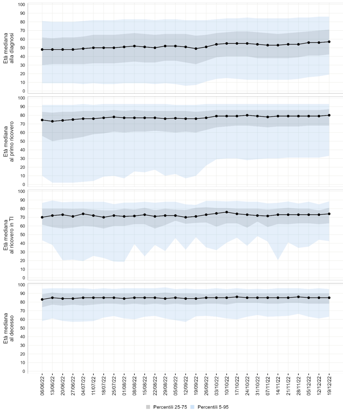
FIGURA 7 - ETÀ MEDIANA DEI CASI DI INFEZIONE DA SARS-CoV-2 ALLA DIAGNOSI, AL PRIMO RICOVERO, AL RICOVERO IN TERAPIA INTENSIVA E AL DECESSO IN ITALIA PER SETTIMANA DI DIAGNOSI
