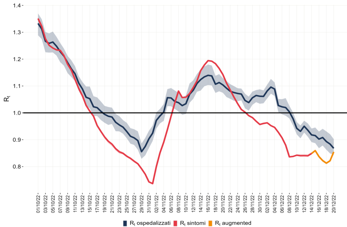
FIGURA 17 - ANDAMENTO GIORNALIERO DI R_t SINTOMI, R_t OSPEDALIZZAZIONI E R_t AUGMENTED NAZIONALE, CALCOLATO IL 28 DICEMBRE 2022
