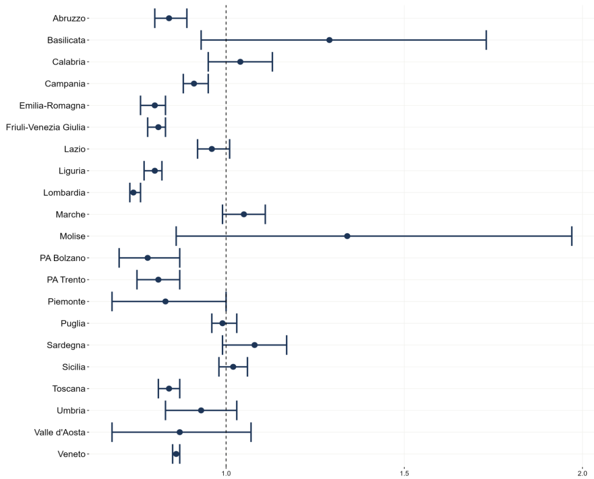
FIGURA 18 - STIMA DELL'RT SINTOMI AL 14 DICEMBRE 2022 CALCOLATO IL 28 DICEMBRE 2022 Nota: Per i dettagli vedi Nota Metodologica paragrafo 2
