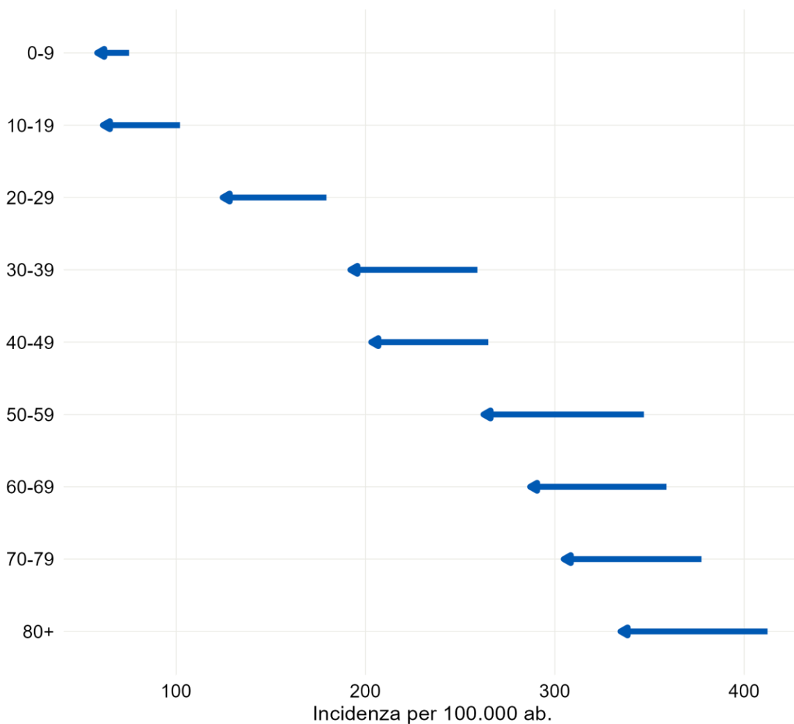
FIGURA 16 - ANDAMENTO DEL NUMERO DI INFEZIONI DA SARS-CoV-2 (PER 100.000 AB.) SEGNALATE PER FASCIA DI ETÀ NEL PERIODO 19 - 25 DICEMBRE 2022 RISPETTO AL NUMERO SEGNALATO DAL 12 - 18 DICEMBRE 2022
