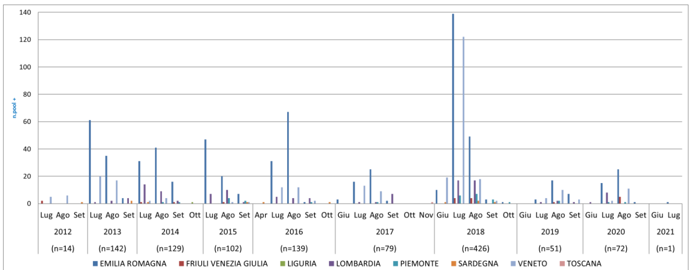
Figura 3 Andamento spazio-temporale della presenza del WNV nelle zanzare catturate - 2021
