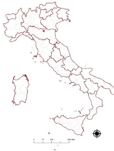
Figura 2 Distribuzione geografica dei pool di zanzare risultate positive nei confronti del WNV - 2021
