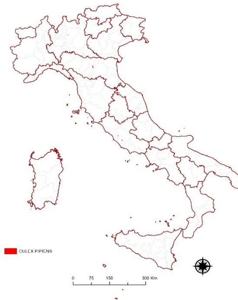
Figura 4 Distribuzione geografica dei pool di zanzare ed uccelli risultati positivi nei confronti dell'USUV - 2021
