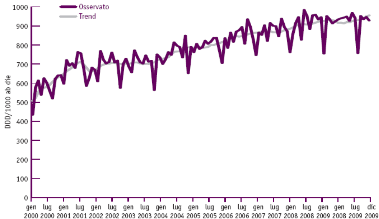
Figura A.3 Andamento del consumo territoriale ^ di classe A-SSN (2000-2009)
