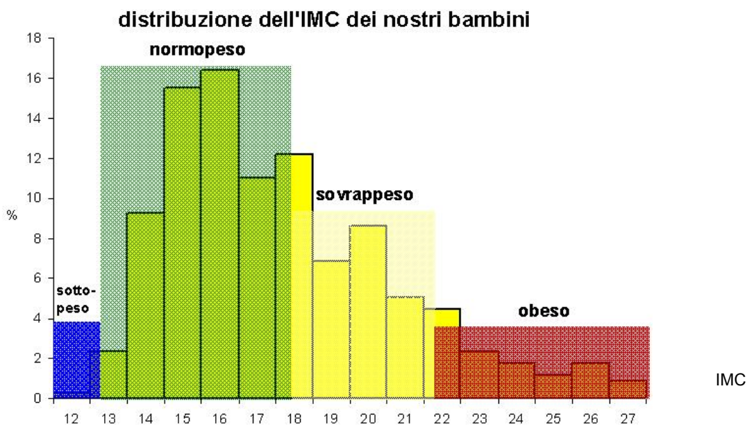
Fig. 2 L'istogramma rappresenta la distribuzione dei bambini in rapporto allo stato nutrizionale del 2010: sotto-normopeso, sovrappeso, obesi (analisi limitata ai bambini dell'età mediana della popolazione in studio a livello nazionale +/- 6 mesi: da otto anni e quattro mesi a nove anni e quattro mesi); n = 336 Non si riscontrano differenze di rilievo tra le due curve.
