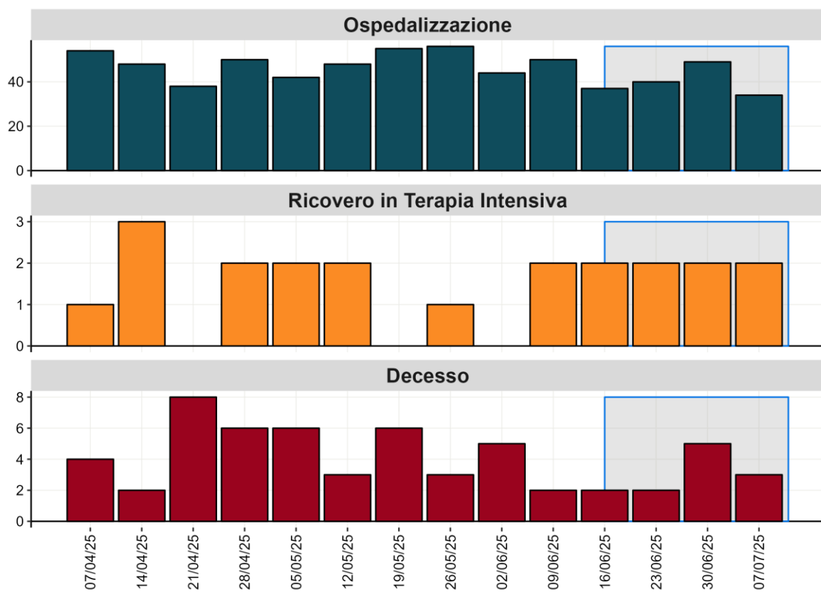
Figura 11 - Numero settimanale di ospedalizzazioni, ricoveri in terapia e decessi per settimana dell'evento a partire dal 7 aprile 2025
