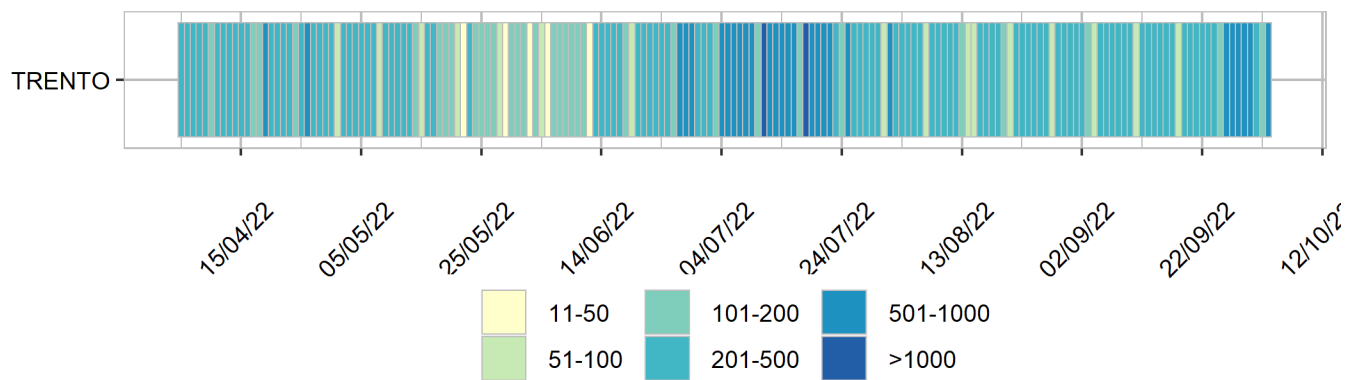
Heatmap - casi
