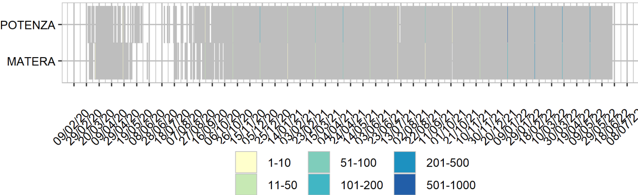
Heatmap - casi
