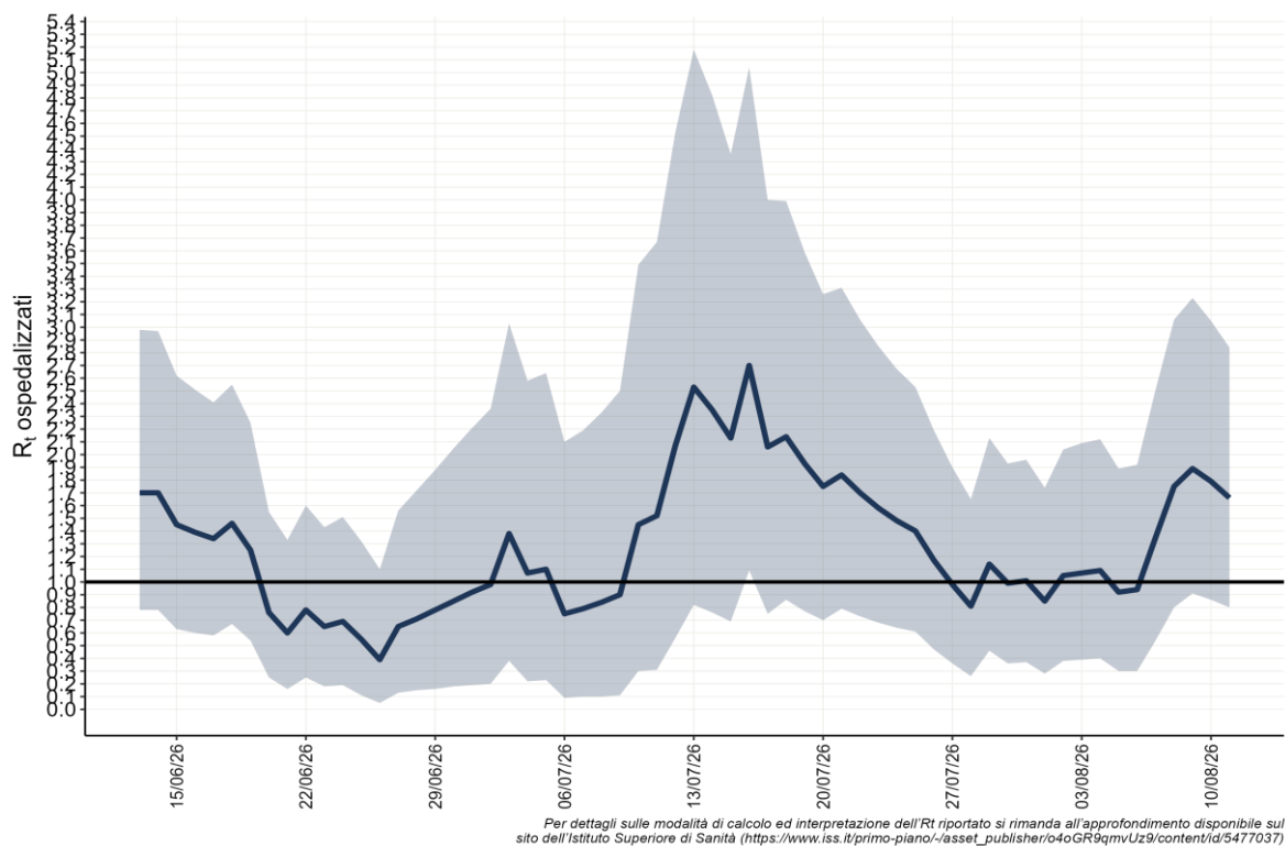
Figura 8 - Andamento giornaliero di Rt ospedalizzazioni nazionale, calcolato con dati estratti il 19 agosto 2026
